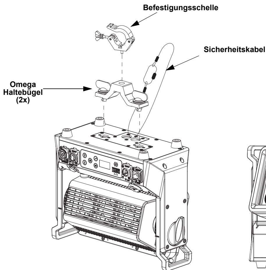
Montage über Kopf
