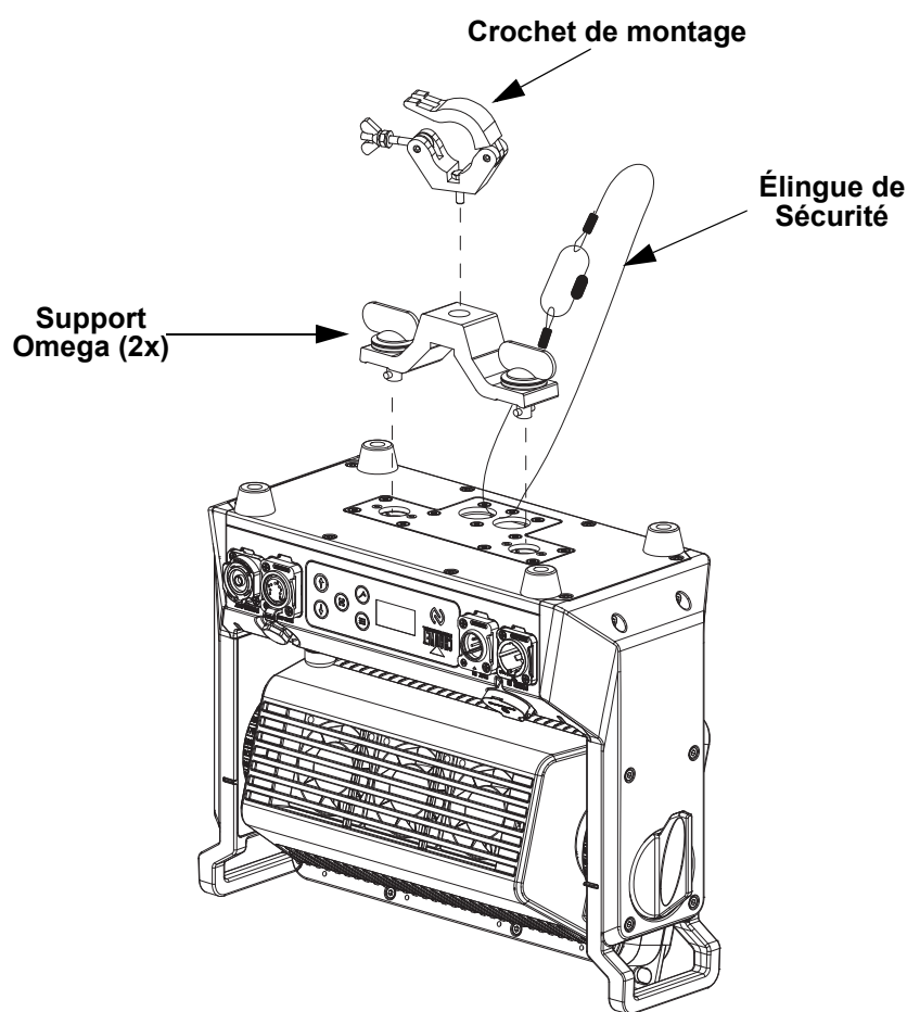
Montage en hauteur
