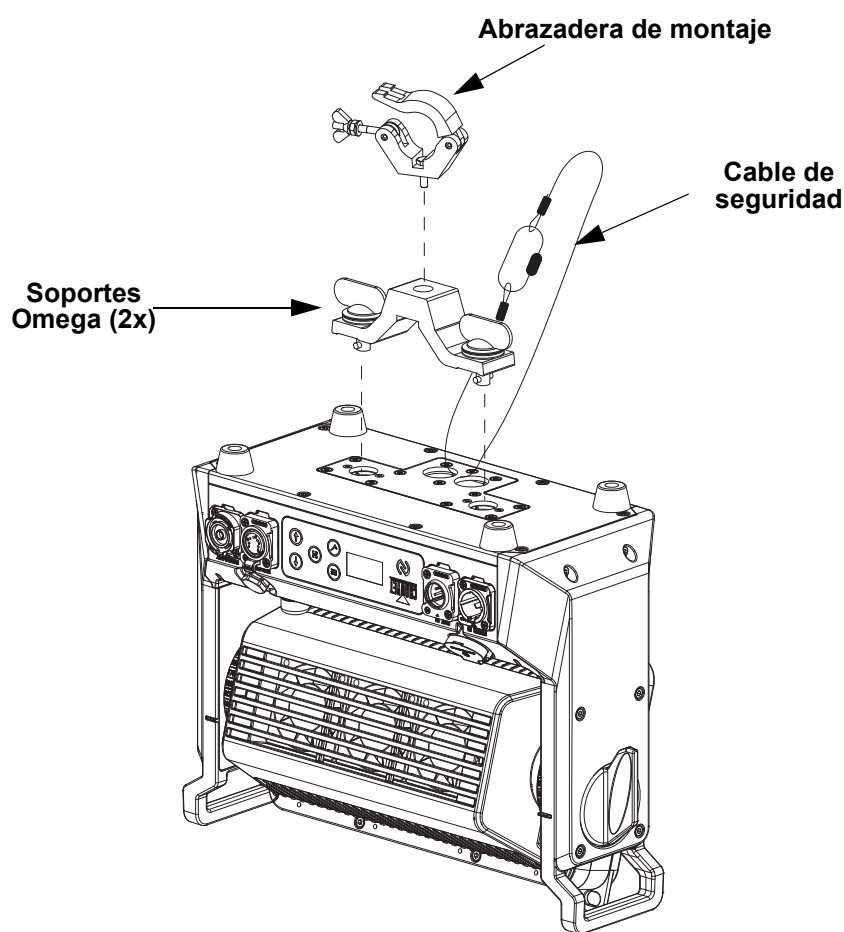
Montaje en altura
