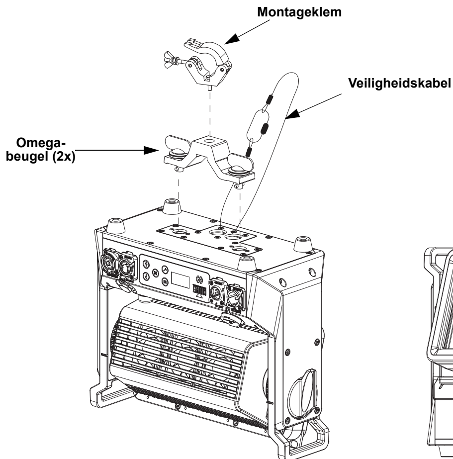
Montage boven het hoofd
