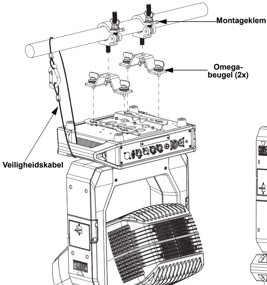
Montage boven het hoofd
