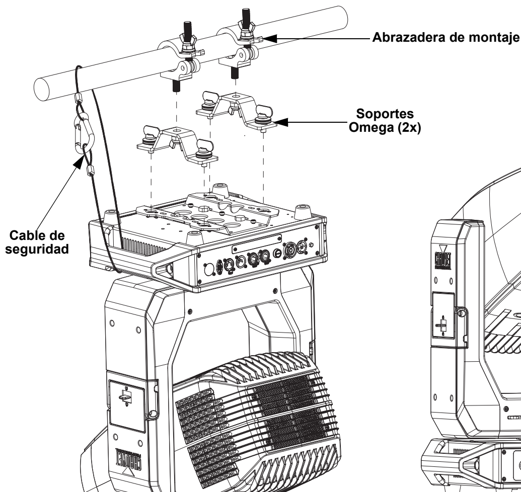
Montaje en altura
