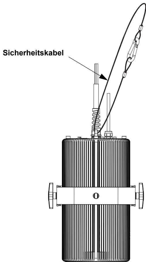
Montageansicht
