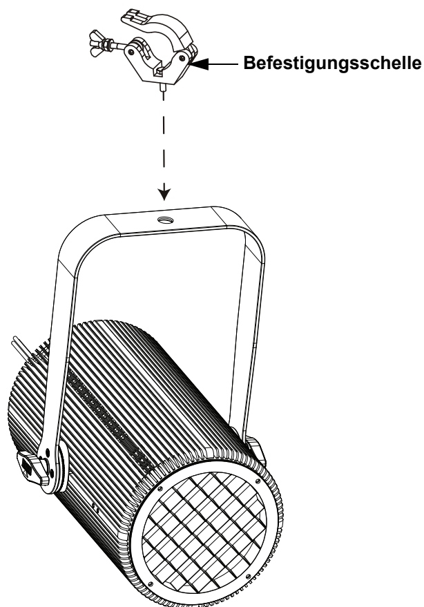
Hängende Montage
