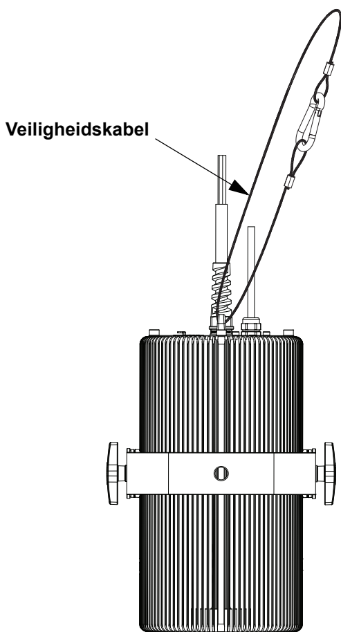
Pendelmontage
